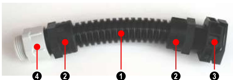
Abbildung 1: Wellschlauch WS21/150
