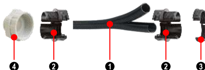
Abbildung 3: Einzelteile des Sets Wellschlauch WS21/150
