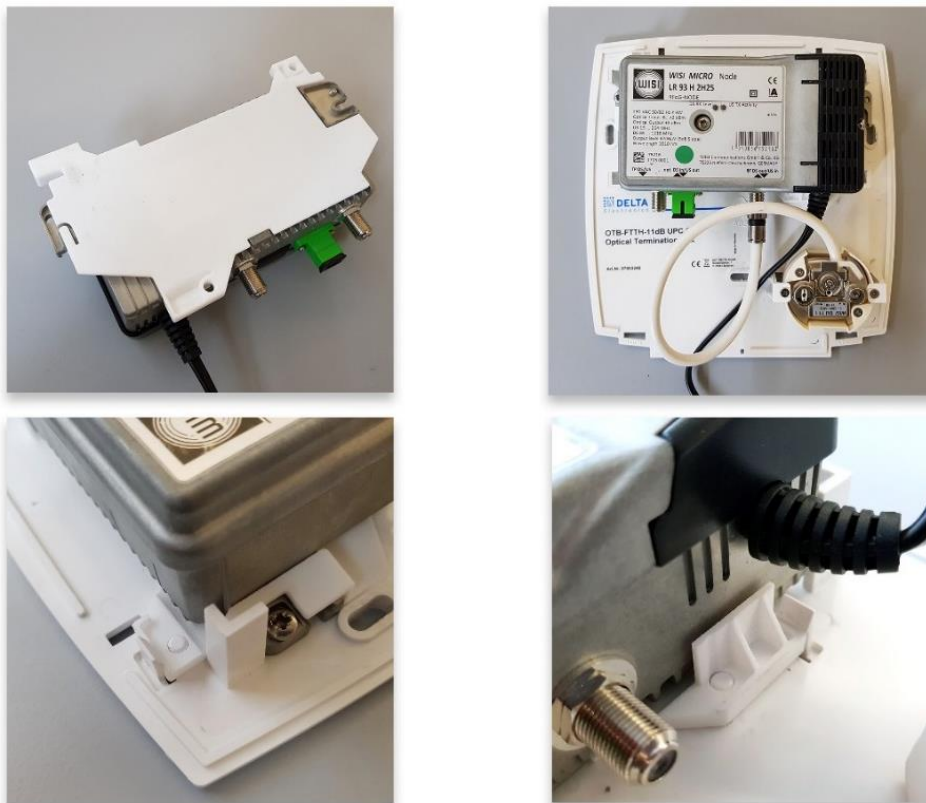
Abbildung 1: Adapterplatte LZ93 für Einbau in FTTH Micronode Abdeckung ONHA23, Delta
